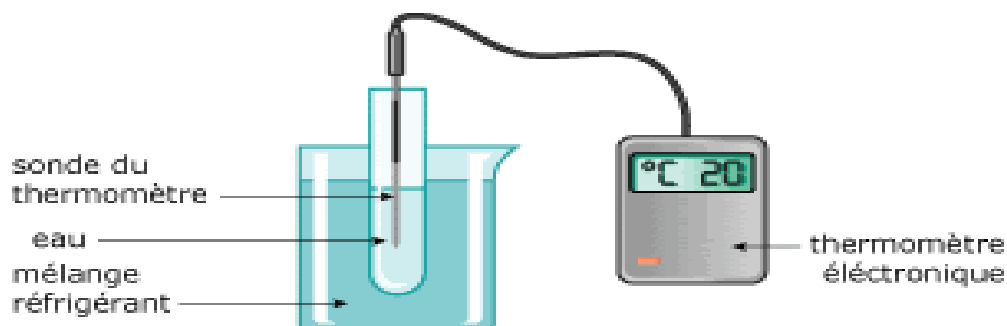
Figure II.2 : Thermomètre électronique [9].
