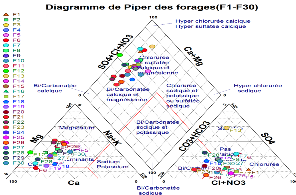
Figure V.14 : Classification des Forages (1-30) sur diagramme de PIPER
