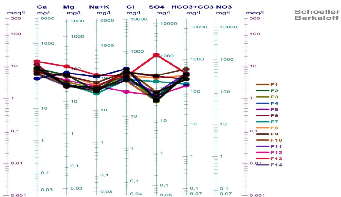
Figure V.16 : Représentation des résultats d'analyses (F1-F14) selon le diagramme de Schoeller-Berkaloff
