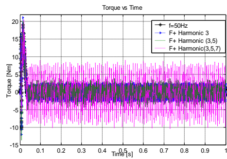
a. Sinusoidal
