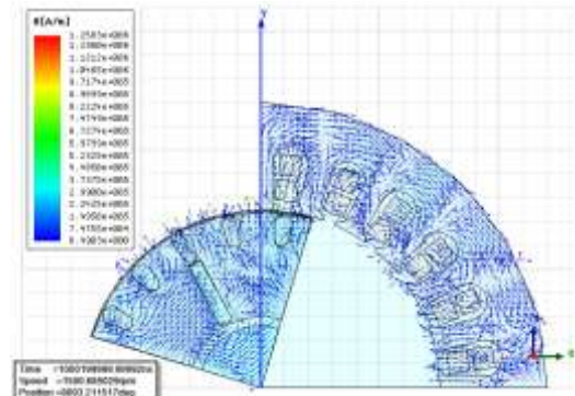
a. Sinusoidal
