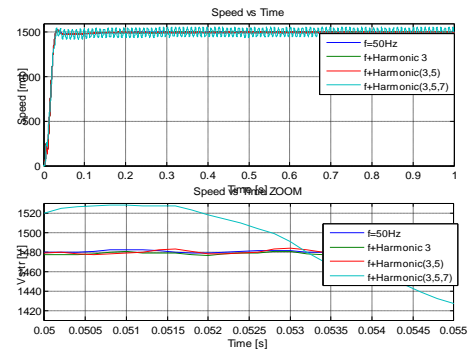
a. Sinusoidal
