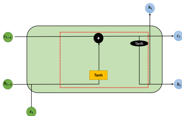
FIGURE 4.6 – Architecture d'une Cellule LSTM [ Basé sur [6] ]
