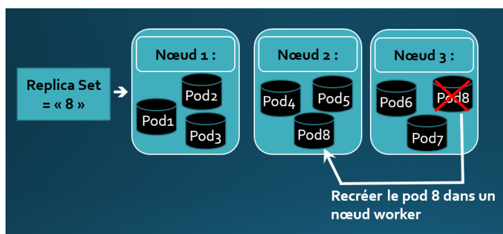
FIGURE 3.3 – Architecture de Réplicasets [ Basé sur [22] ]
