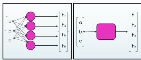
FIGURE 4.2 – Architecture des MLP [ Basé sur [58] ]
