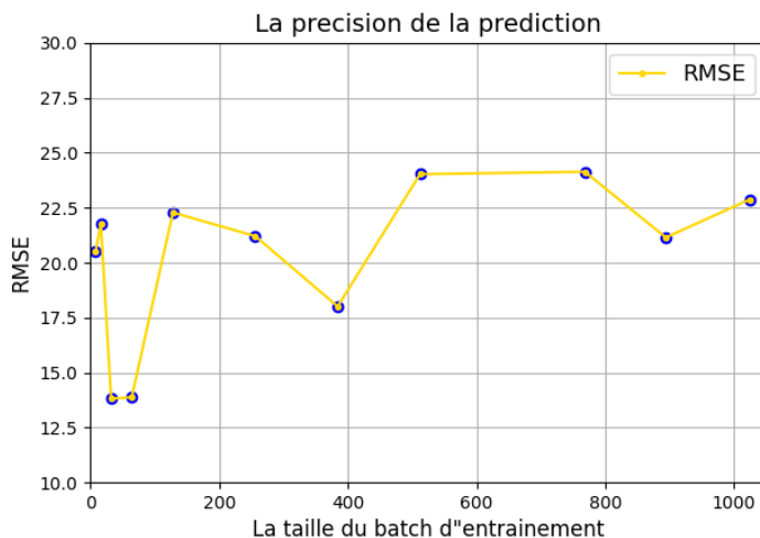
FIGURE 7.2 – RMSE Globale pour Chaque Valeur de Batch size
