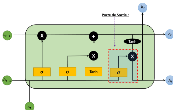
FIGURE 4.10 – Représentation de la Porte de Sortie [ Basé sur [6] ]
