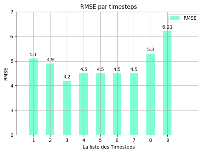
FIGURE 7.11 – RMSE par TimeSteps avec la Meilleure Taille de la Fenêtre de Prédiction
