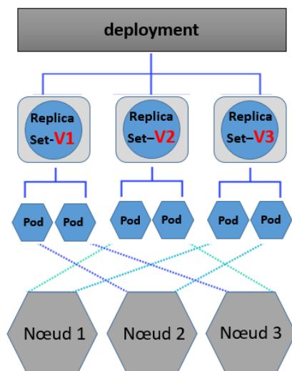
FIGURE 3.4 – Déploiement [ Basé sur [22] ]
