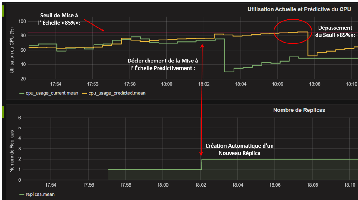
FIGURE 7.14 – Démonstration de MEAP en Utilisant "Grafana"
