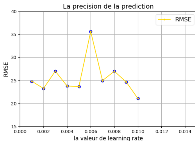
FIGURE 7.12 – RMSE Globale en Changeant la Valeur du taux d'apprentissage (Learning Rate \alpha )
