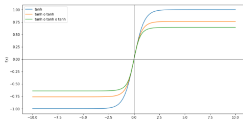
FIGURE 4.4 – Passages Successifs sur la Fonction Tangente Hyperbolique [51]
