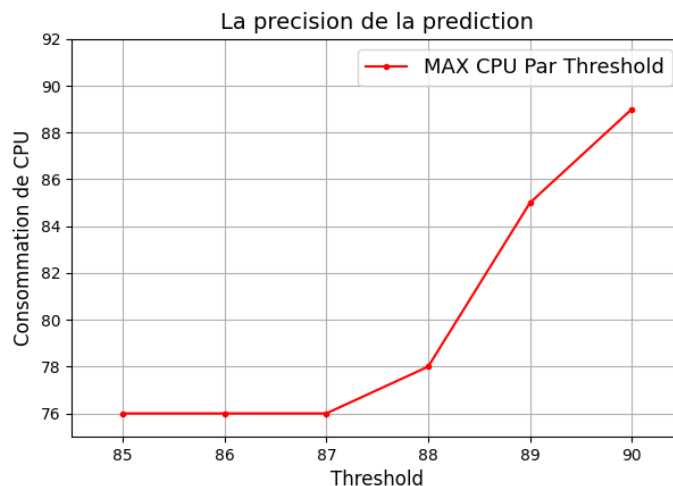
FIGURE 7.15 – Maximum consommation de CPU en variant la valeur du seuil de mise à l'échelle qu'on doit tester, ce qui motive à laisser cette question ouverte pour qu'elle soit traitée comme perspective.
