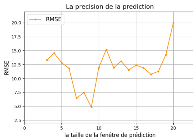
FIGURE 7.10 – RMSE Globale pour Chaque Taille de la Fenêtre de Prédiction (TimeSteps)
