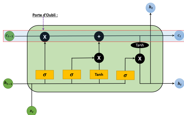
FIGURE 4.9 – Représentation de l'État de la Cellule [ Basé sur [6] ]
