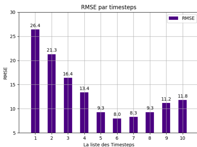
FIGURE 7.5 – RMSE par TimeSteps avec le meilleur nombre d'époques
