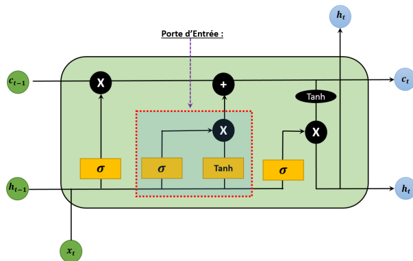
FIGURE 4.8 – Présentation de la Porte d'Entrée [ Basé sur [6] ]
