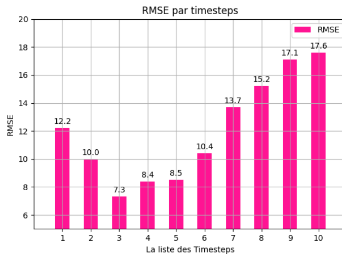
FIGURE 7.9 – RMSE par TimeSteps avec la meilleur taille du vecteur h
