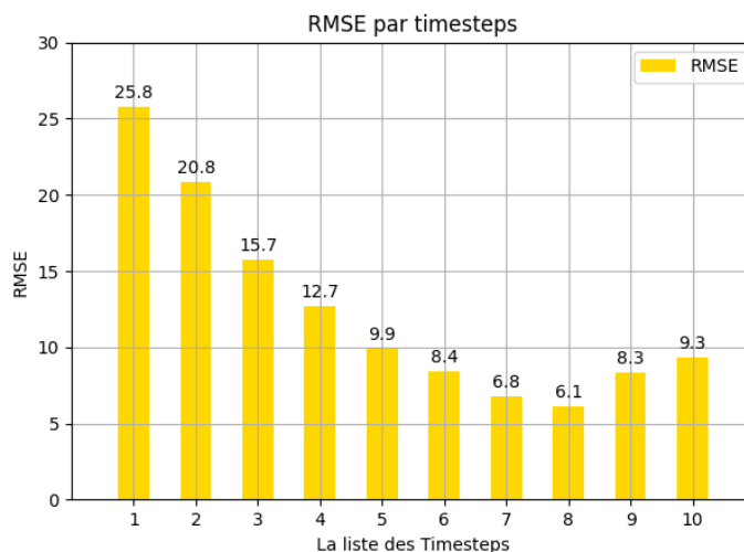
FIGURE 7.3 – RMSE par TimeSteps avec la Meilleur Batch Size
