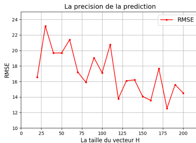
FIGURE 7.8 – RMSE Globale pour Chaque Taille du Vecteur h
