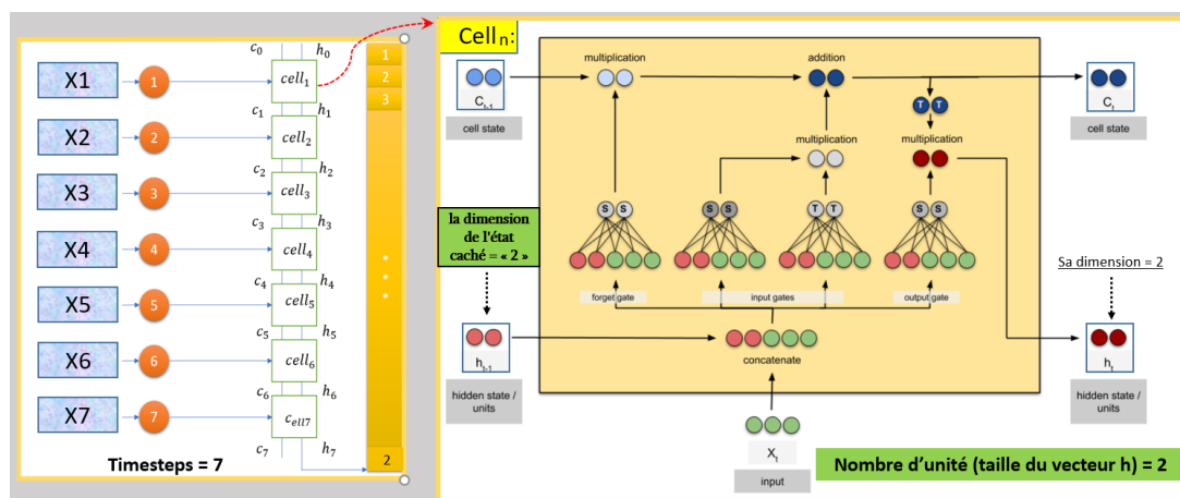
FIGURE 4.21 – Nombres d'unités en LSTM [ Basé sur [44] ]
