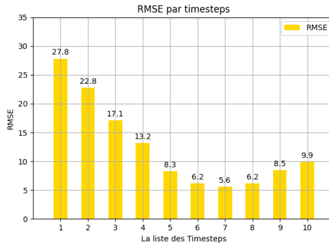
FIGURE 7.7 – RMSE par TimeSteps avec la Meilleur Batch Size
