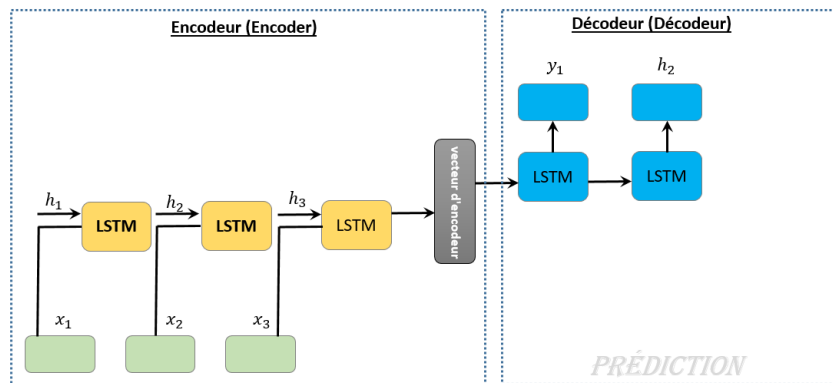
FIGURE 4.19 – Architecture du Modèle Encodeur-Décodeur [ basé sur [50]]
