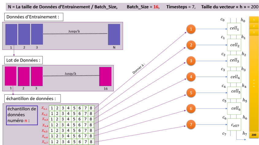
FIGURE 4.22 – Le Batch Size (Taille du Lot) [ Basé sur [11] ]
