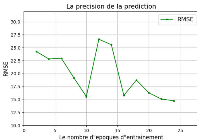
FIGURE 7.4 – RMSE Globale Pour Chaque Valeur d'époque
