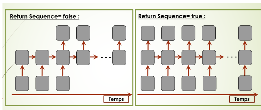
FIGURE 4.15 – Plusieurs à Plusieurs (Many-to-Many) [ Basé sur [59] ]
