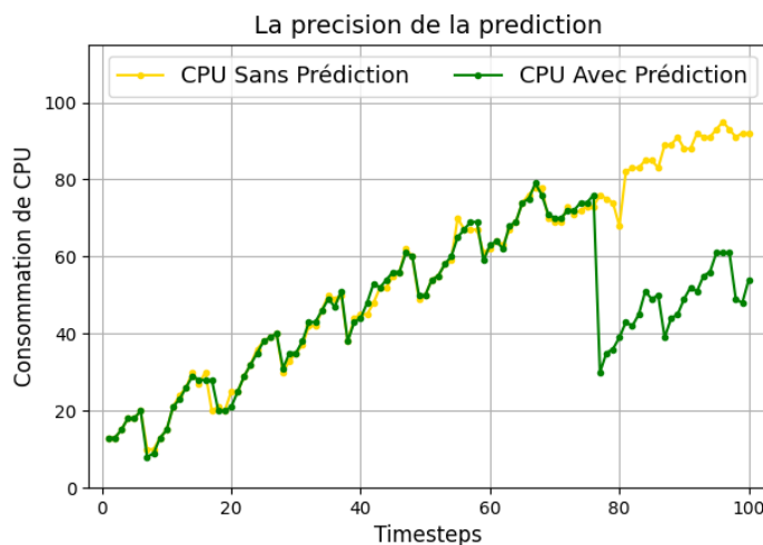
FIGURE 7.13 – Comparaison de la consommation de CPU en utilisant l'approche de mise à l'échelle automatique et prédictive et l'approche de mise à l'échelle automatique non prédictive
