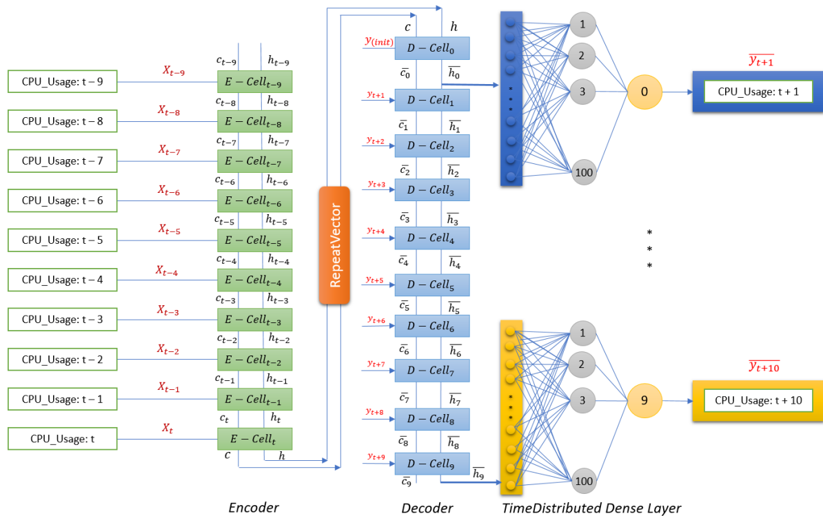
FIGURE 6.2 – Architecture du Modèle de Prédiction Utilisé ( LSTM Encodeur-Décodeur)
