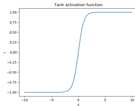
FIGURE B.2 – La Fonction Tanh, [31]
