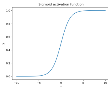
FIGURE B.1 – La Fonction Sigmoid [31]
