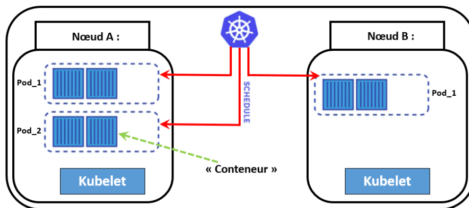
FIGURE 3.2 – Architecture d'un Pod [ Basé sur [67] ]
