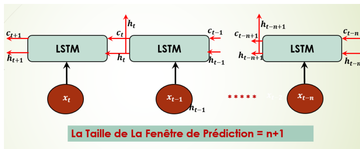
FIGURE 4.20 – La Fenêtre de Prédiction (TimeSteps) [ Basé sur [75] ]
