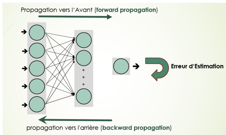
FIGURE 4.11 – Rétro-propagation du gradient [ Basé sur [69] ]
