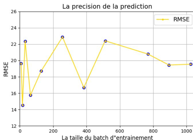
FIGURE 7.6 – RMSE Globale pour Chaque Valeur de Batch Size avec le Meilleur Nombre d'époques Trouvé
