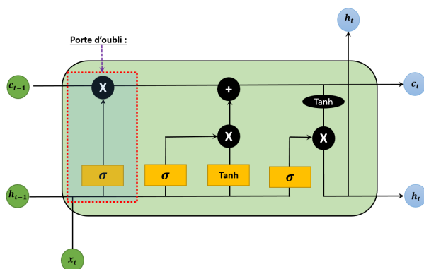
FIGURE 4.7 – Représentation de la porte d'oubli [ Basé sur [6] ]
