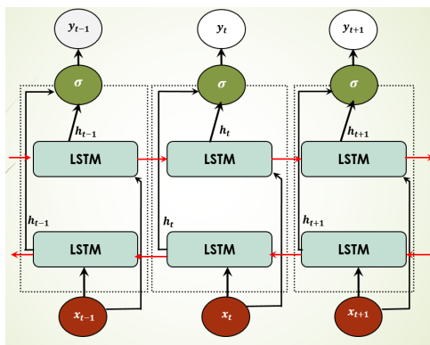
FIGURE 4.17 – Architecture de LSTM Bidirectionnels [ Basé sur [12]]
