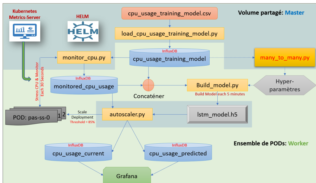
FIGURE 7.1 – Plateforme de Mise à l'Échelle Automatique et Prédictive
